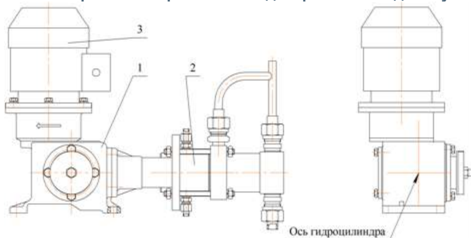
Рис. 1 - Агрегат электронасосный дозировочный одноплунжерный дифференциальный
