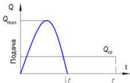
График подачи простого одностороннего насоса
