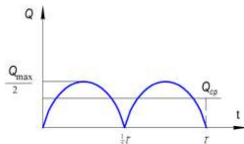
График подачи дифференциального насоса
