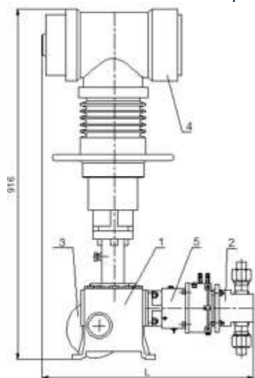
Рис. 1 - Насос дозировочный одноплунжерный герметичный
