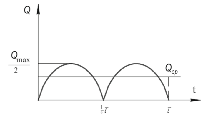
Рис.2.25 Графики подачи простого одностороннего и дифференциального насосов
