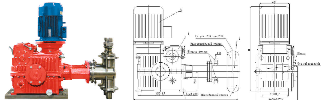
Рис.2.13 Агрегат серии AP44 одноплунжерный с гидроцилиндром одностороннего действия
