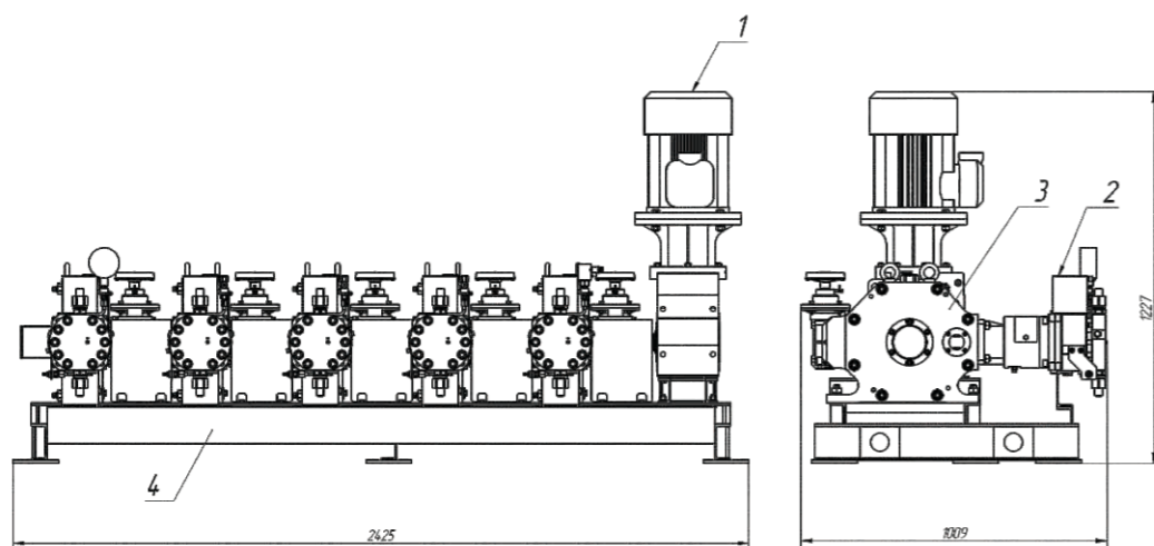
Строение блочного агрегата серии АР45 Рис.3.8
