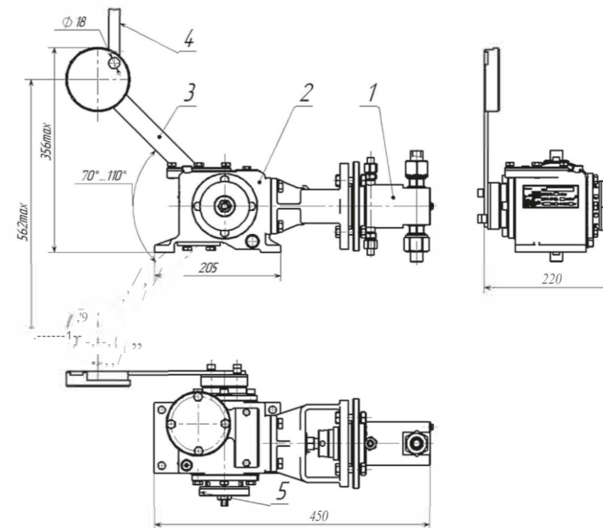
Рис 4.1 Насос дозирочный плунжерный типа НД с приводом от станка-качалки
